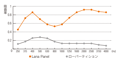
■ 残響室法吸音率測定より
